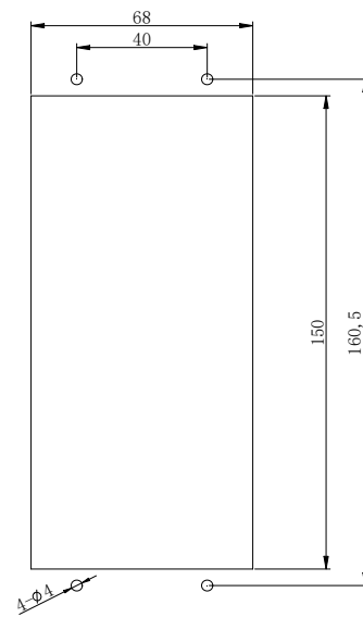
开孔尺寸
